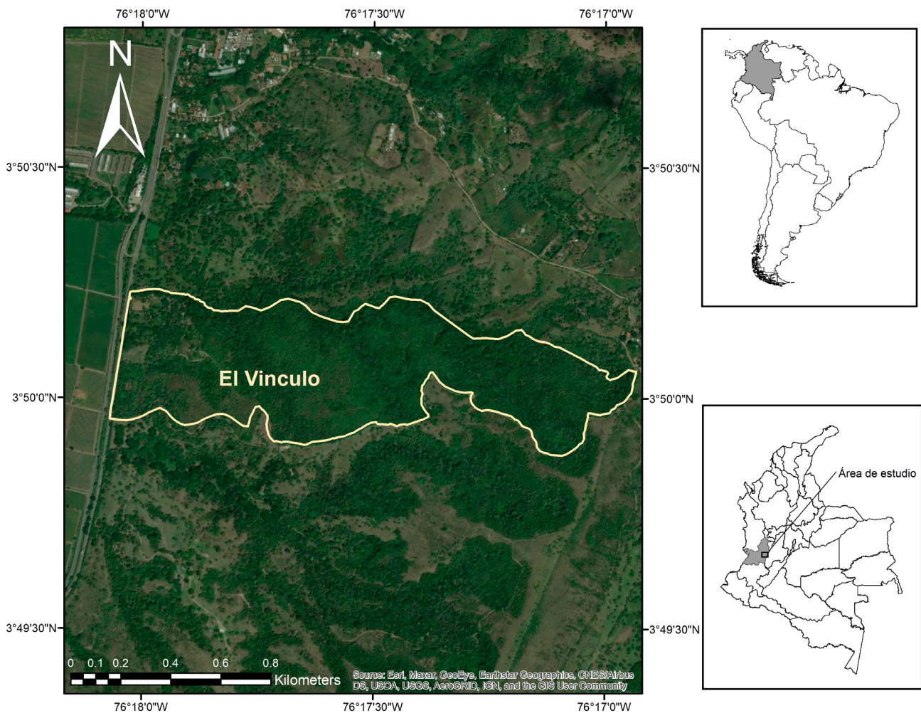
Figura 1. Parque Natural Regional El Vínculo, Buga, Valle del Cauca, Colombia. Figure 1. El Vínculo Regional Natural Park, Buga, Valle del Cauca, Colombia.
