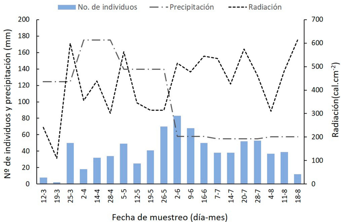
Figura 5. Número de individuos de mariposas Ithomiini por fecha de captura (día-mes), para las dos temporadas climáticas, y su respectiva precipitación mensual promedio (mm) y radiación diaria (cal.cm -2 ), en el Parque Natural Regional El Vínculo, Buga, Colombia. Temporada de lluvias: marzo, abril y mayo. Temporada seca: junio, julio y agosto.
